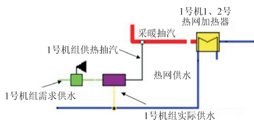
图2 12号控制器调节热网加热器工况 [31]
