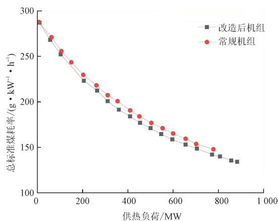
图5 THA 工况机组总标准煤消耗量变动情况 [32]
