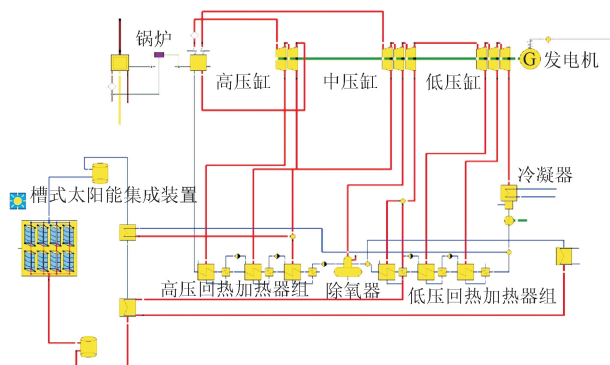
图 11 300 MW 太阳能辅助热电联产系统 [63]
