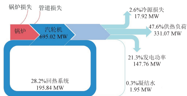
图 8 切缸工况能流图 [47]
