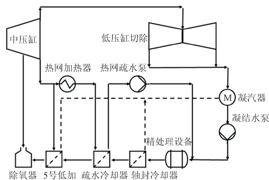
图6 轴封冷却器和加热器之间布置方案 [43]
