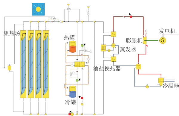
图13 槽式太阳能热发电回热循环系统模型 [67]
