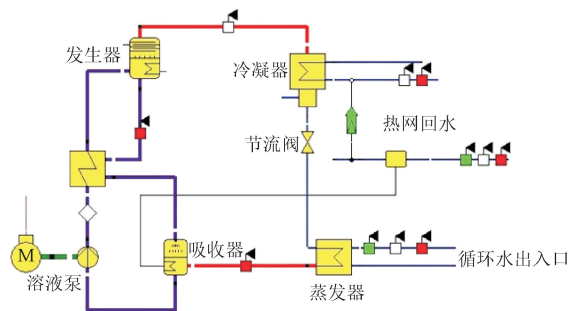
图1 耦合吸收式热泵系统图 [29]
