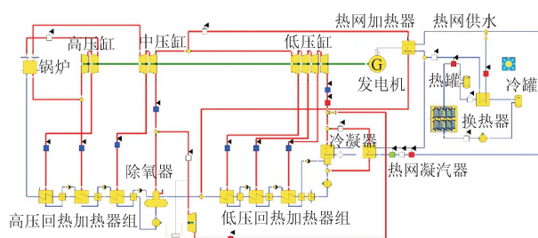
图 12 基于 EBSILON 的太阳能辅助抽气采暖改造机组 [66]
