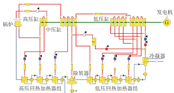
图 10 使用 EBSILON 软件搭建 350 \text{ MW} 模型 [57]
