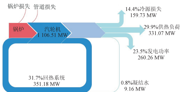
图 7 抽汽供热工况能流图 [47]
