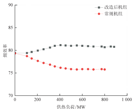
图4 THA 工况下汽水系统烟效率变化 [32]
